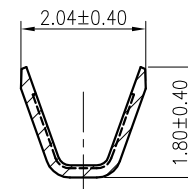
SECTION B-B SCALE 2:1
